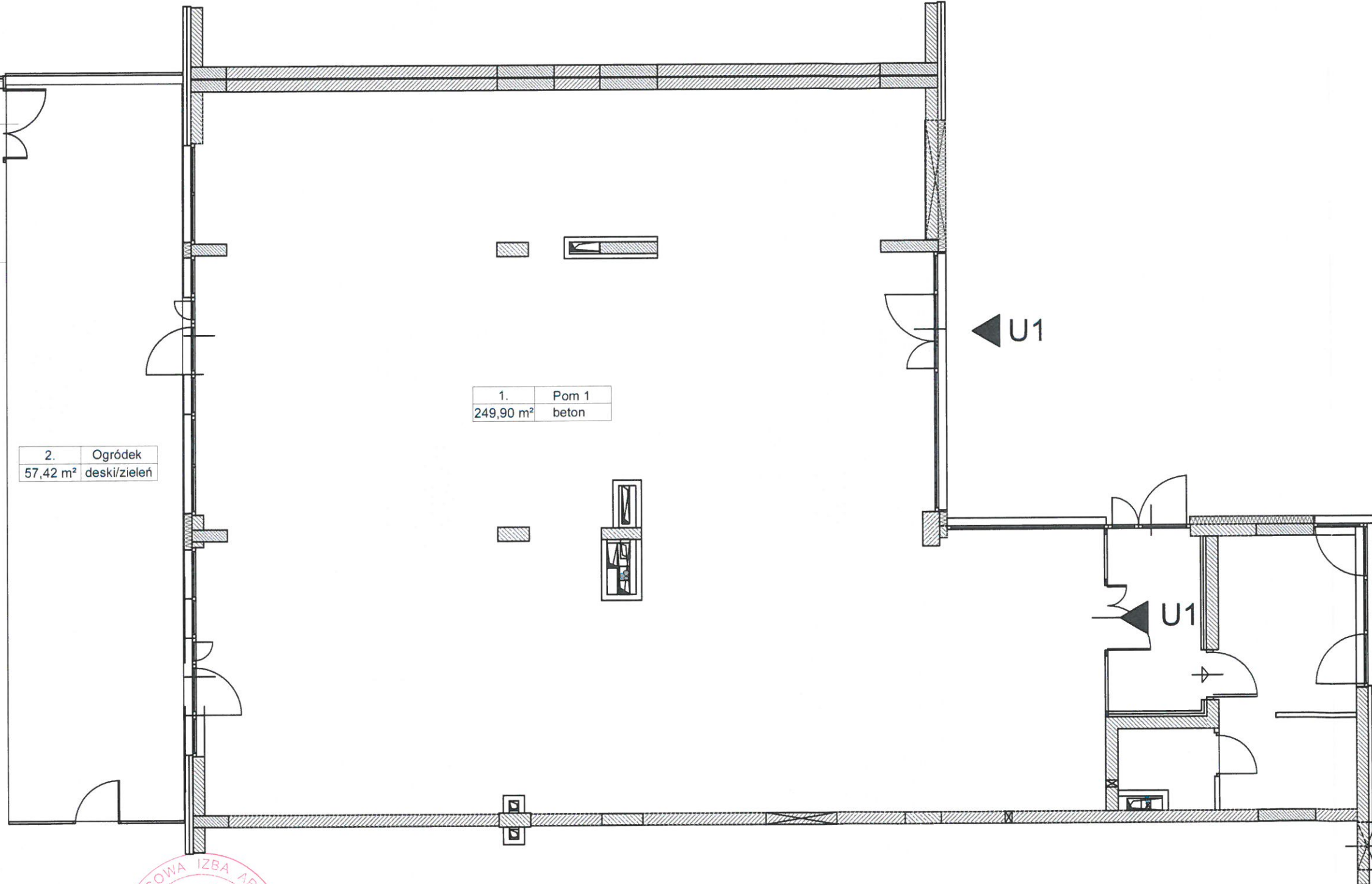
Schemat kondygnacji
